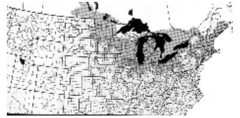
Range Map
